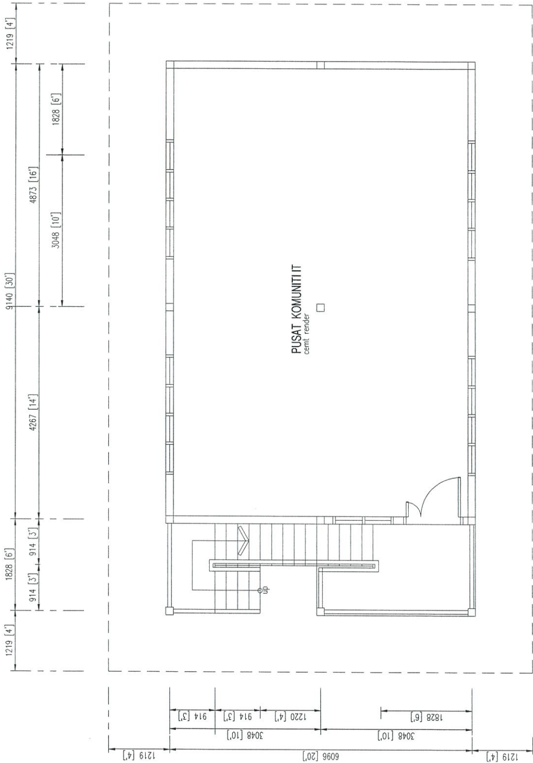
PELAN TINGKAT SATU SKALA 1:75 BALAIRAYA SEK. 17/1A
