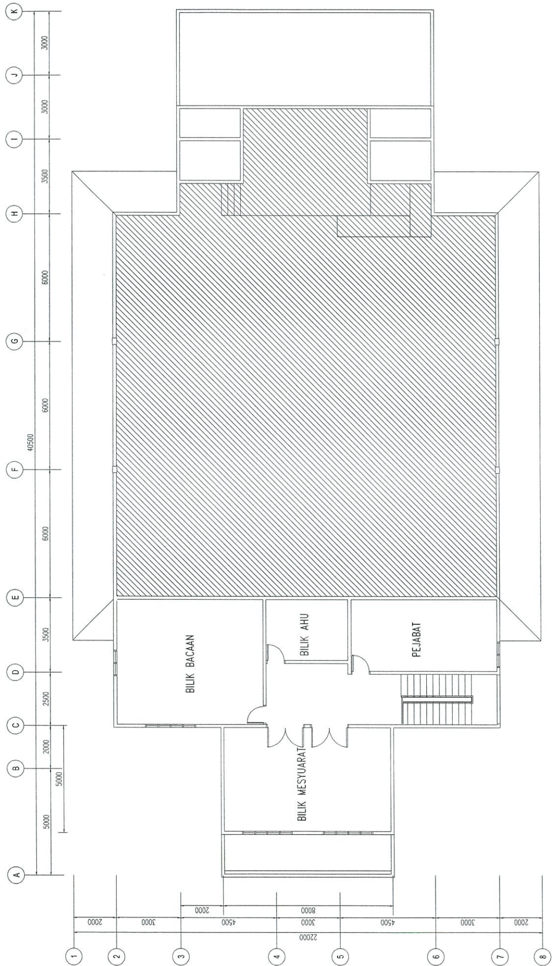
PELAN LANTAI TINGKAT ATAS SKALA 1 : 175
