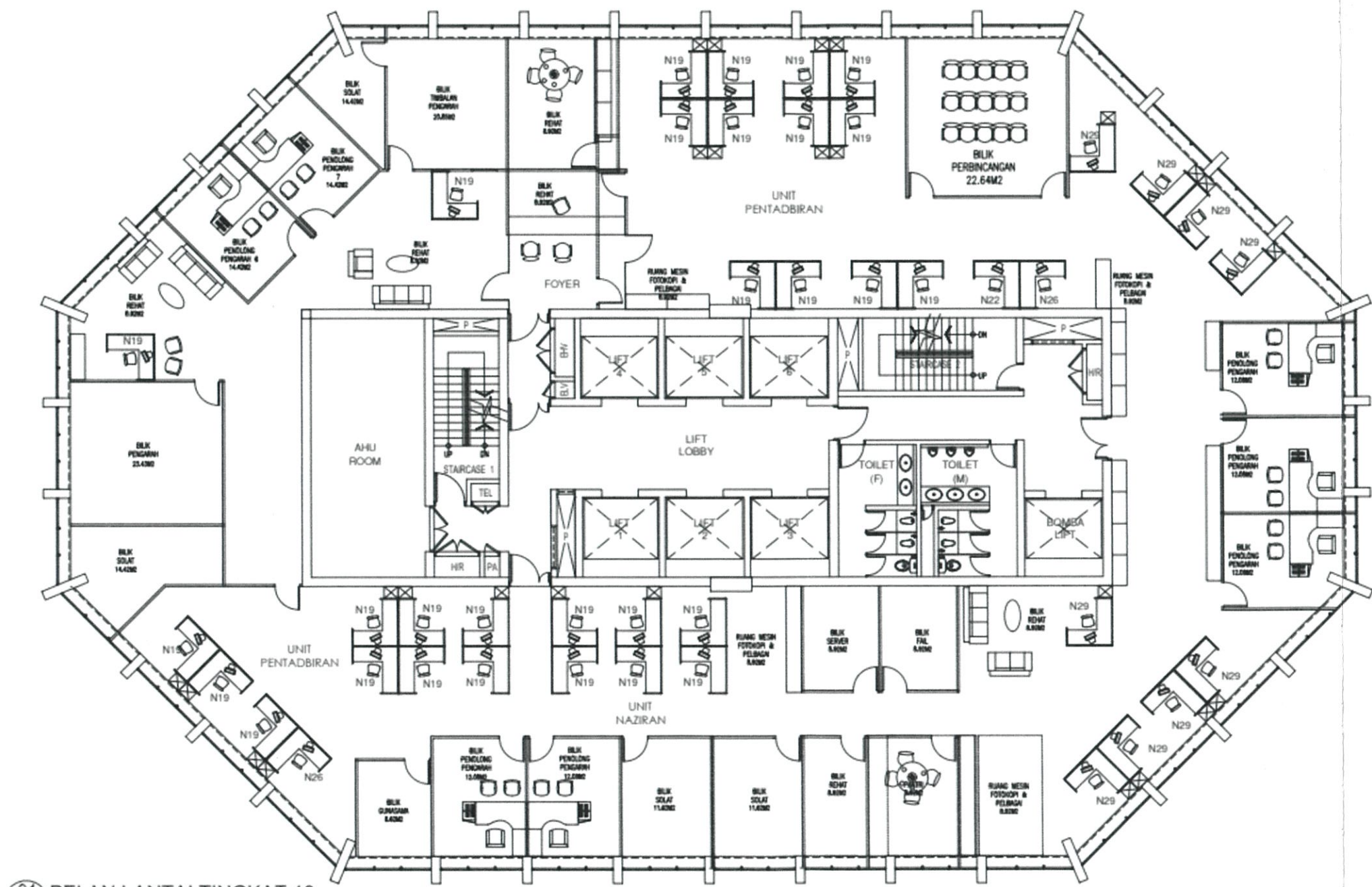
01 PELAN LANTAI TINGKAT 19 100 SKALA = 1 : 100 NET AREA : 820 Sq. Meter GROSS AREA : 1025 Sq. Meter
