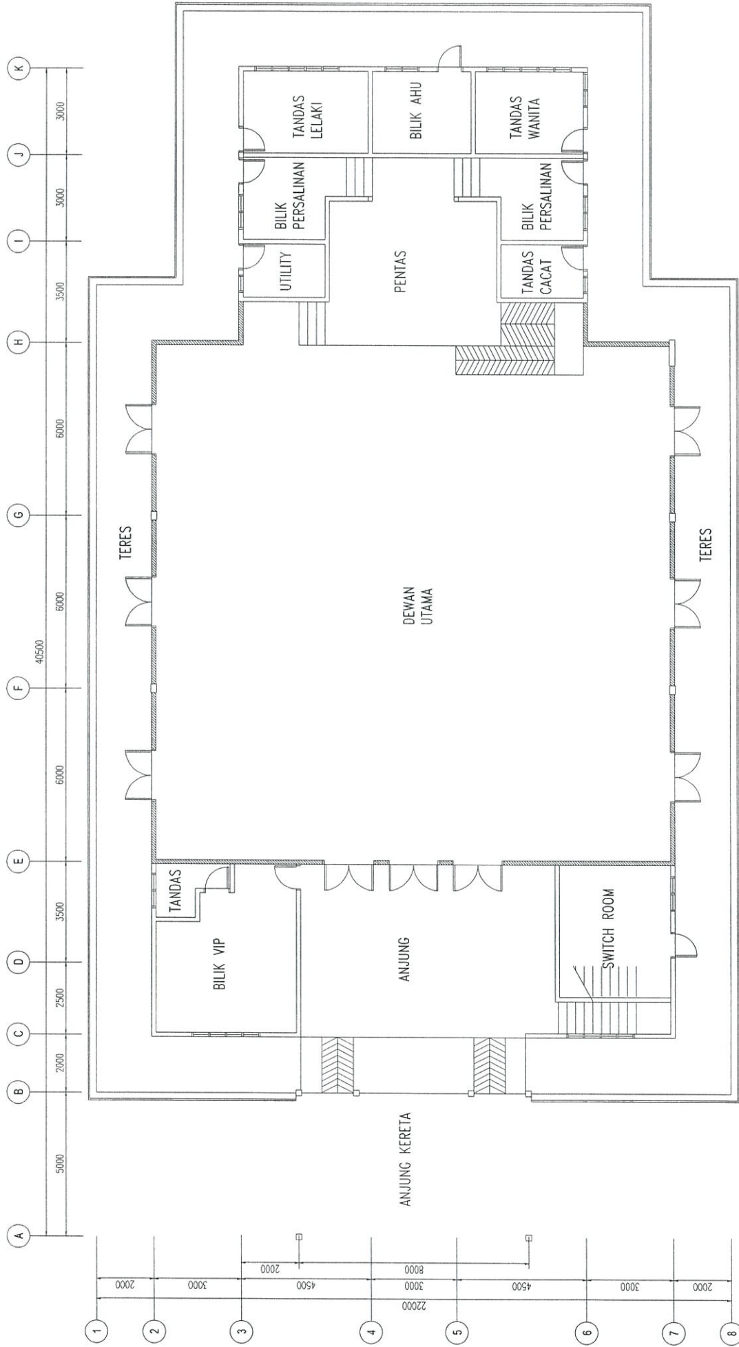
PELAN LANTAI TINGKAT BAWAH SKALA 1 : 175
