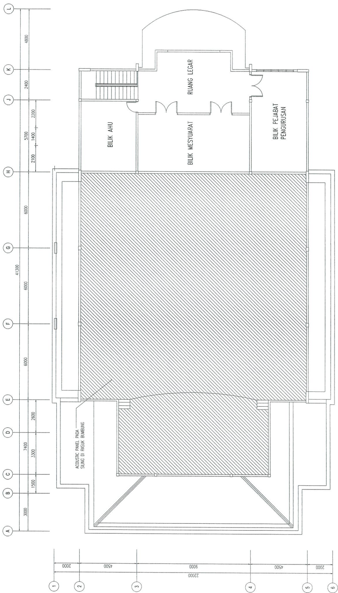
PELAN LANTAI TINGKAT ATAS SKALA 1 : 175 DEWAN SERBAGUNA SRI DAMANSARA, JALAN PERSIARAN PERDANA
