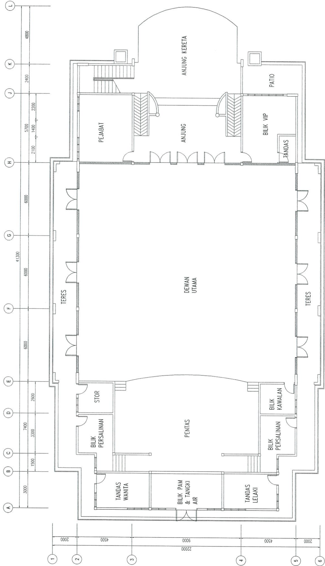
PELAN LANTAI TINGKAT BAWAH
