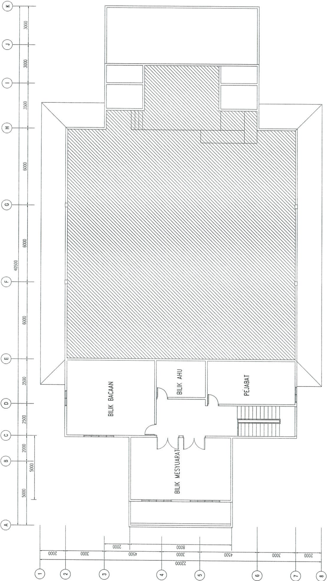
PELAN LANTAI TINGKAT ATAS SKALA 1 : 175 DEWAN SERBAGUNA PERSIARAN MAHOGANI, JALAN SD 1/3, SRI DAMANSARA
