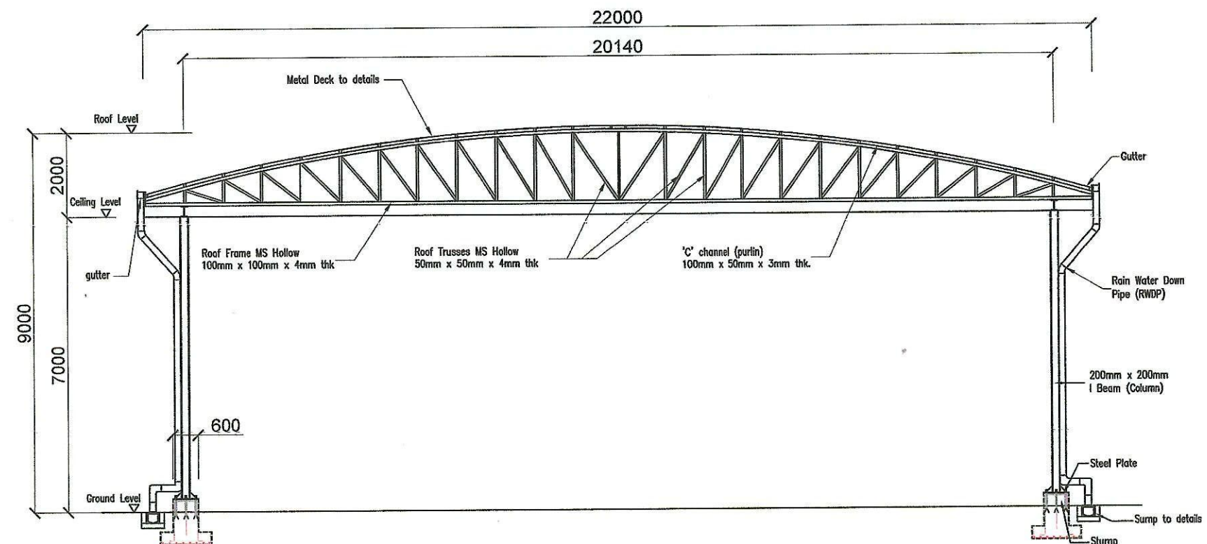
SECTION A-A
